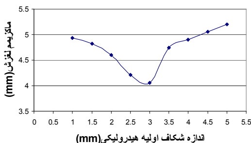
شکل ۸ تغییرات شاخص گسیختگی در مقابل اندازه شکاف اولیه (برای دسته درزه‌های متعامد +90^\circ و 0^\circ درجه)
