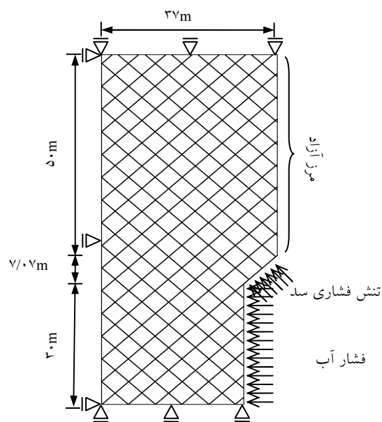
شکل ۳ تکیه‌گاه شبیه سازی شده
