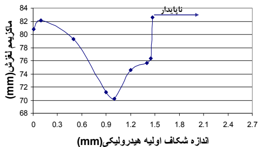
شکل ۷ تغییرات شاخص گسیختگی به ازای تغییر اندازه شکاف اولیه (برای دسته درزه‌های متعامد +45^\circ و -45^\circ درجه)
