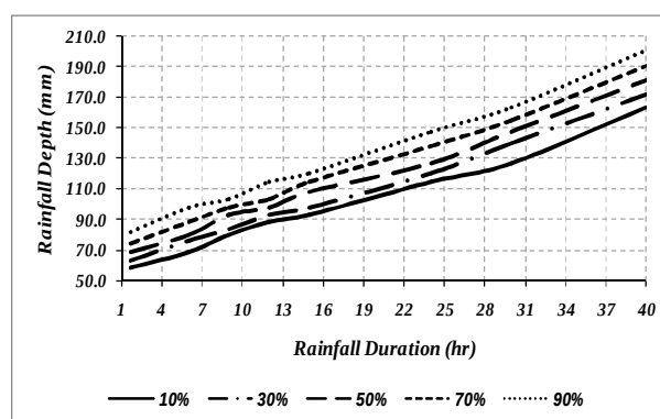
شکل 7 منحنی بارش آستانه روگذری سد جامیشان
