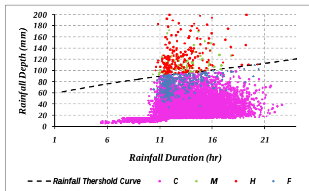
شکل 9 تقسیم‌بندی وقایع بر اساس منحنی بارش آستانه لبریز شدن
