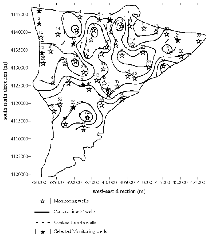
شکل 4 مقایسه منحنی‌های تراز سطح ایستابی در حالت حذف 9 چاه از شبکه مشاهده‌ای
