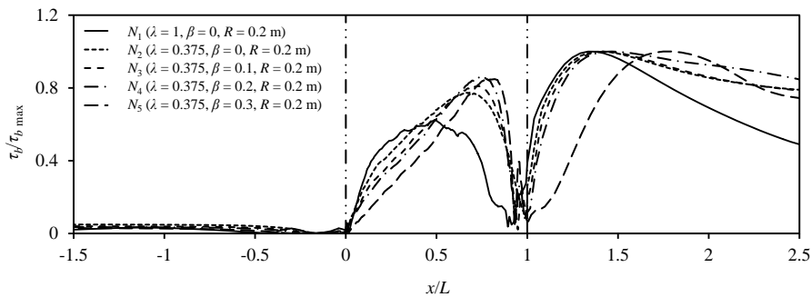
Fig. 14 Dimensionless bed shear stress profiles for different hydrofoil weirs with Q = 70 lit/s شکل ۱۴ نیمرخ‌های بی‌بعد تنش برشی بستر در سرریزهای هیدروفویل مختلف به‌ازای دبی ۷۰ لیتر بر ثانیه
