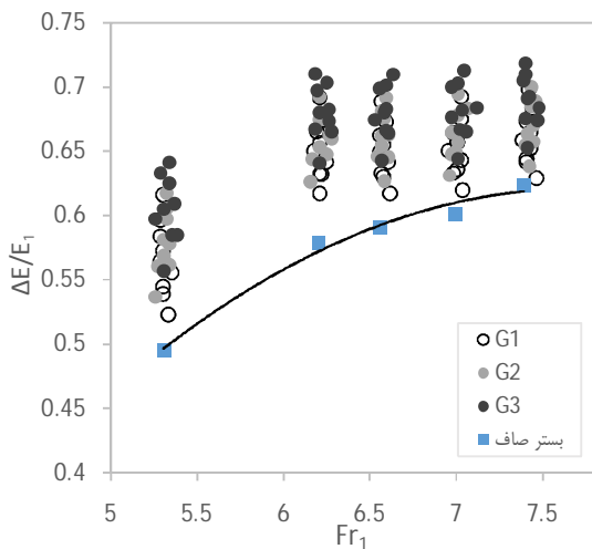
شکل 11 تغییرات افت انرژی نسبی پرش روی بستر نفوذپذیر به ازای عدد فرود اولیه
