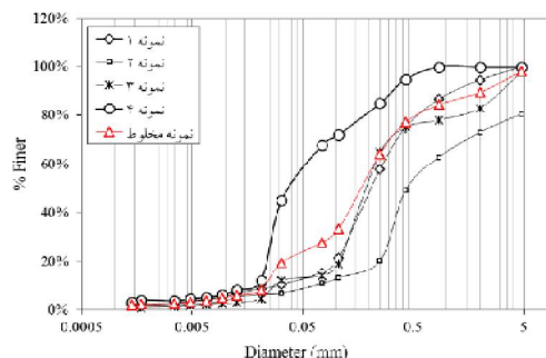
شکل 2 منحنی دانه بندی رسوبات سد کرخه
