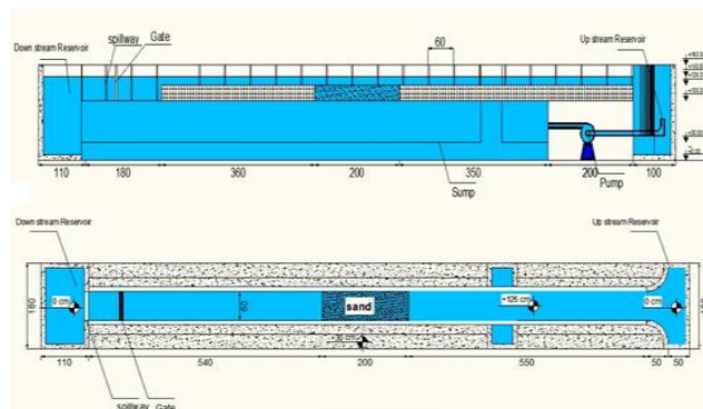
ب- نمای شماتیک از پلان فلوم
