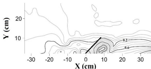
ب) توزیع تنش برشی در مانع میله‌ای دو ردیفه زیگزاگی
