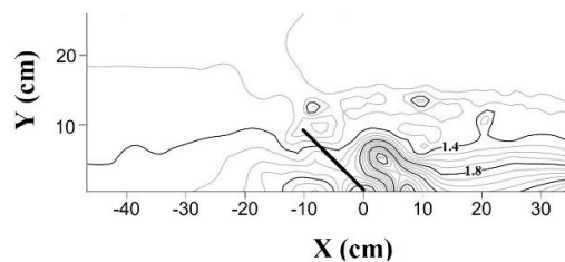
الف) در مانع نفوذناپذیر با زاویه 45 درجه
