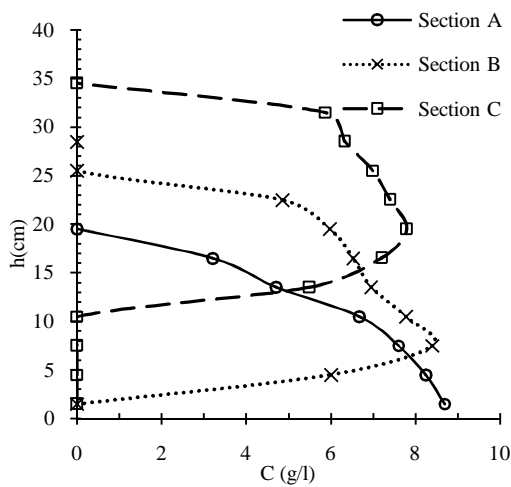
شکل 11 پروفیل غلظت C=10 \text{ g/l} و Q=2.5 \text{ l/s} در سه مقطع مورد آزمایش
