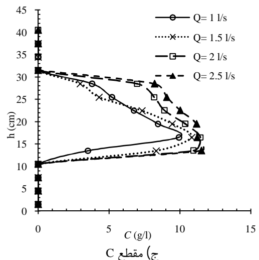
شکل 10 پروفیل غلظت C=15 \text{ g/l}
